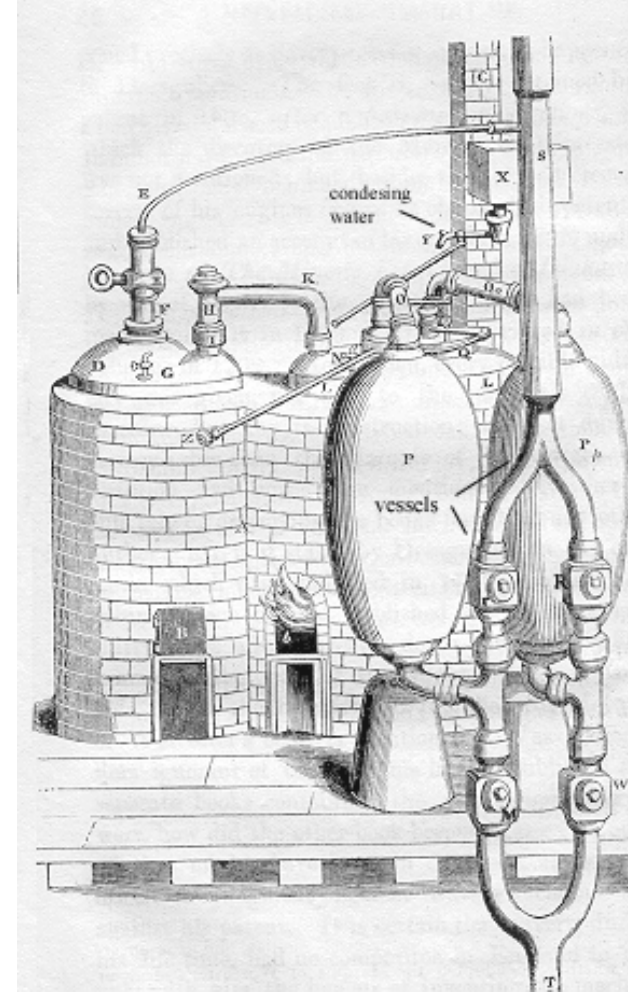
İlk Ticari Buhar Makinesi - 1698
